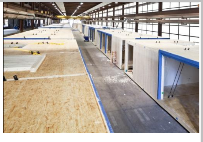
Aneinandergereihte Module in der Montagestrasse
