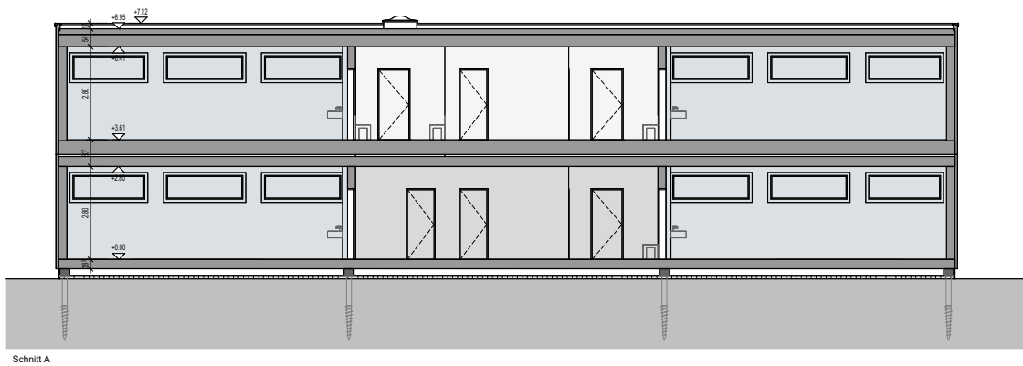
Schnitt A
