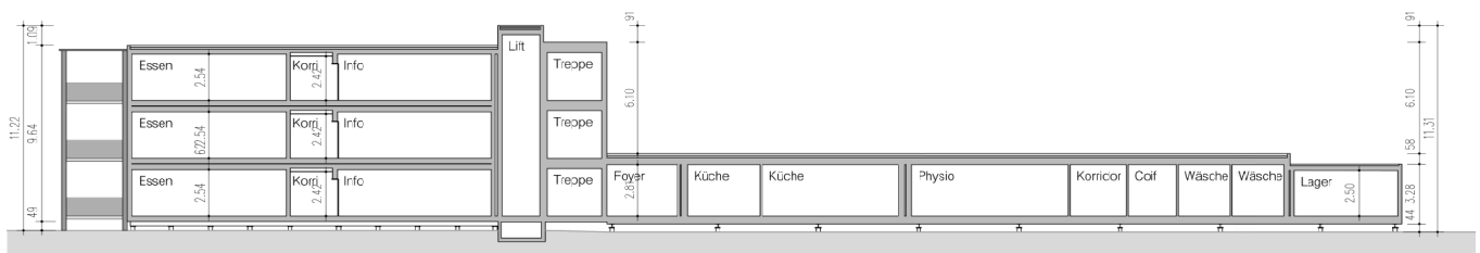
Schnitt
