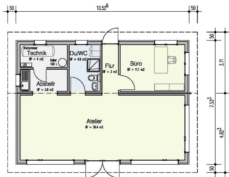
Grundriss
