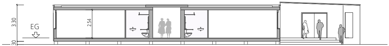
Querschnitt Bettenstation M. 1:200
