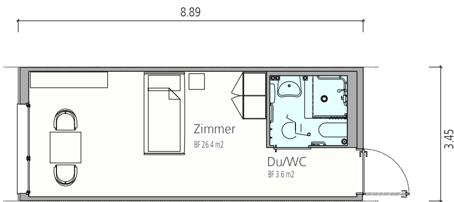
Grundriss Bettenzimmer
