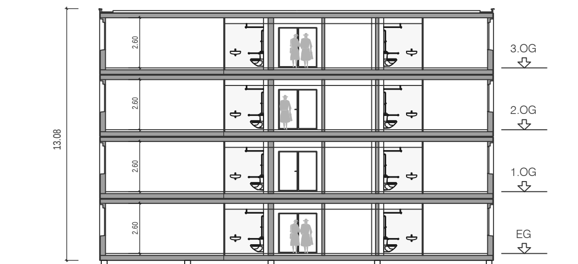
Gebäude- Querschnitt M. 1:200
