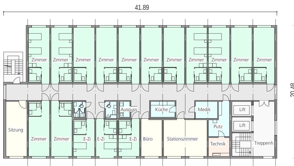
Grundriss 1./2./3.Obergeschoss
